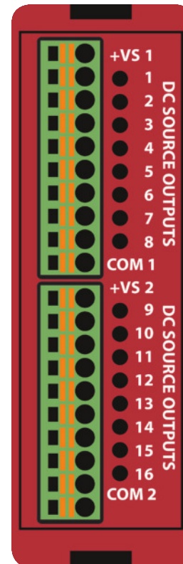
EZRPL-IO-16DCOP
