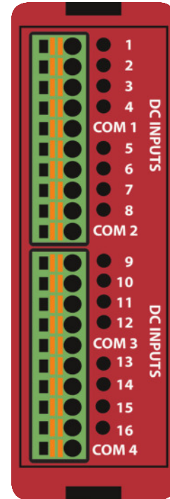
EZRPL-IO-16DCI
