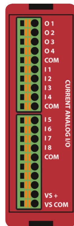
EZRPL-IO-8ANI4ANOC
