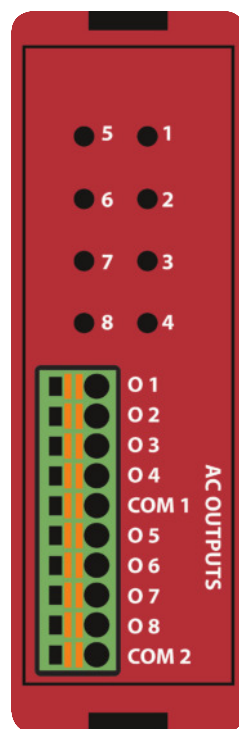
EZRPL-IO-8ACO
