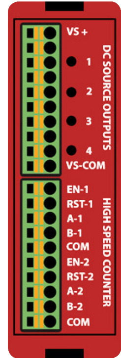
EZRPL-IO-HSCNT
