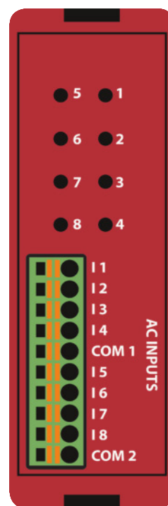
EZRPL-IO-8ACI
